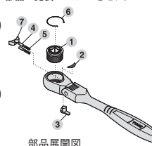
部品展開図
