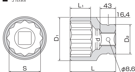
■ 寸法図
