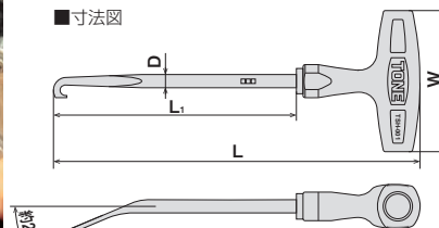
■寸法図
