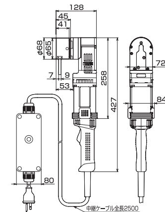
M22用ソケット装着寸法図
