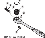
部品展開図
