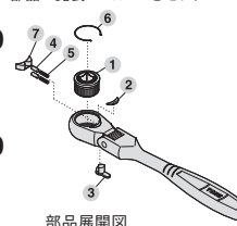
部品展開図
