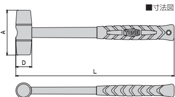
■寸法図
